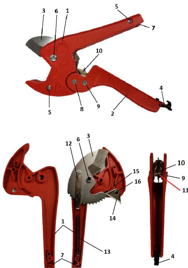
Фото 1. Конструкция ножниц ОТС-42.
