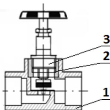
Рис.2 Конструкция вентиля
